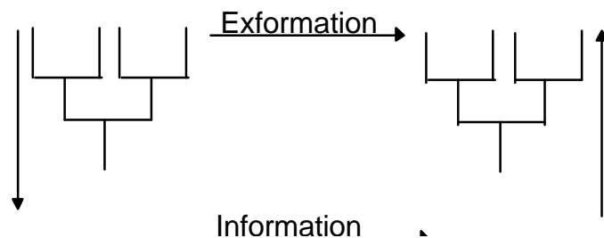
Abbildung 6: Information, Exformation, nach [Norretranders 1994]
