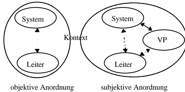
Abbildung 8: objektive und subjektive Masse
